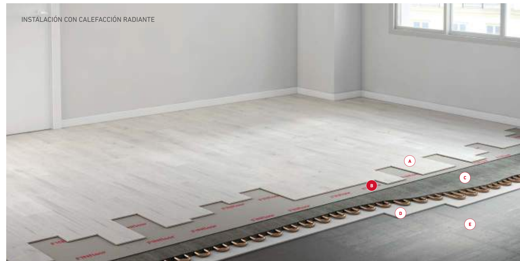
A FINFLOOR B MANTA SILENT ELITE FINFLOOR C CALEFACCIÓN RADIANTE D AISLANTE E SOLERA
