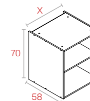
Low Module B70
