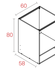
Oven Module B80
